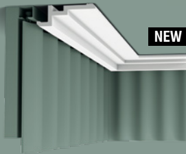
CX196 U-STEPS 200 x 4 x 11,3 cm Duropolymer ®
