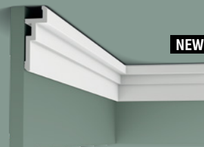
CX196 U-STEPS 200 x 11,3 x 4 cm Duropolymer ®
