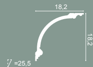
C338B BA'ROCK 200 x 18,2 x 18,2 cm Dessin: 2 x 57 cm Purotouch ®
