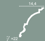
C301 200 x 17 x 14,4 cm Purotouch ®
