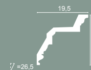
C307 200 x 19,5 x 19,5 cm Purotouch ®
