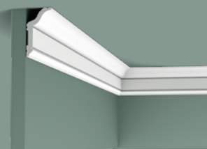
CX141 200 x 5,9 x 3,1 cm Duropolymer ®
