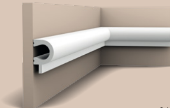
PX169 A 200 x 5,5 x 3,4 cm Duropolymer®
