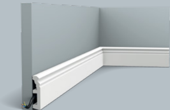
1 SX195 | SX195F HAMBURG 200 x 8 x 1,9 cm Duropolymer ®
